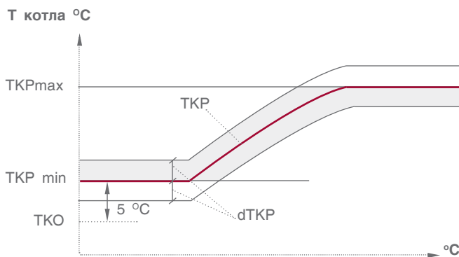
График 2. Граница задания уставки номинальной температуры котла
