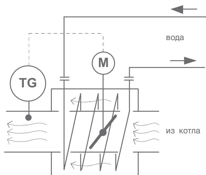
Экономайзер
