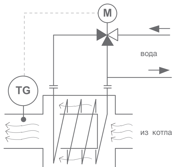
Экономайзер
