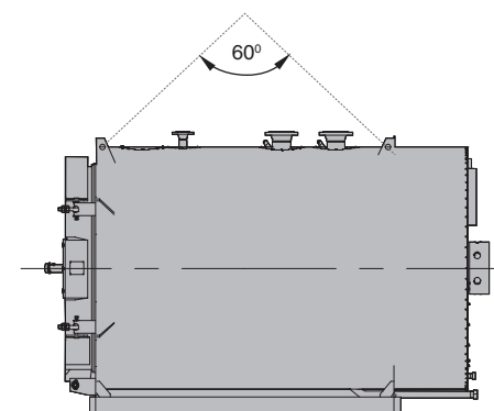
Рис. 7 Принципиальная схема строповки котла
