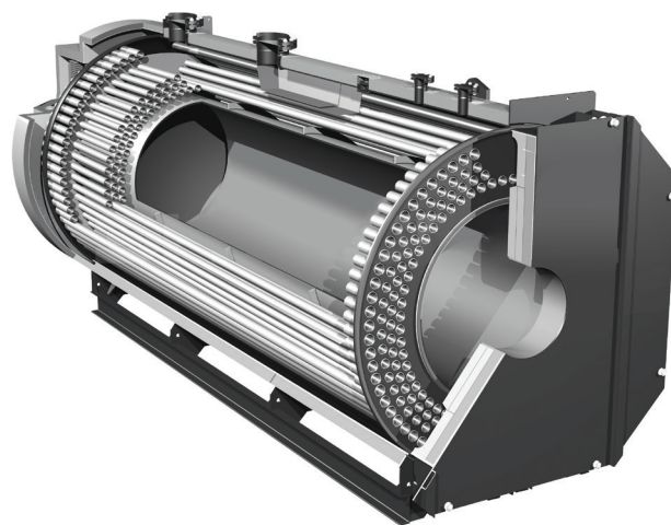
Рис. 1. Общий вид котла ТТ 100-01
