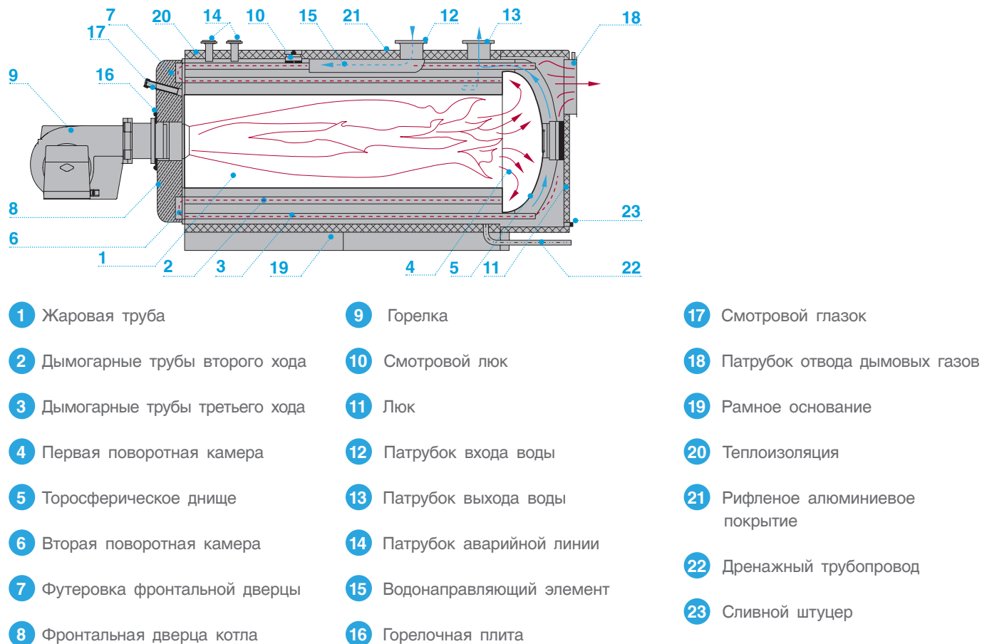
Рис. 2 Принципиальная схема работы котла ТТ100-01
