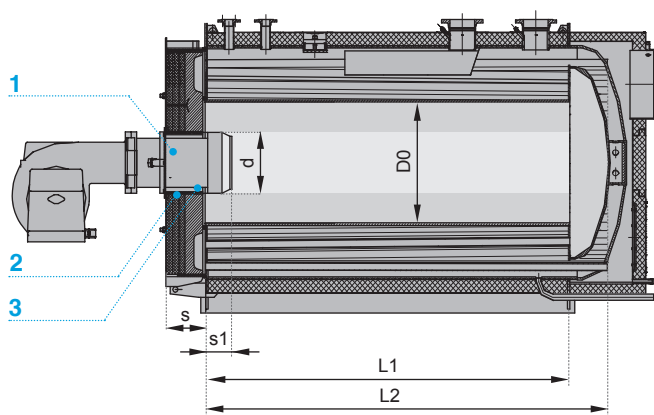
Рис. 5. Установка горелки
